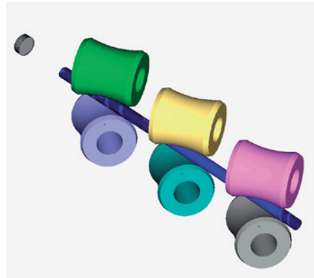
Simulation von Schrägwalzrichten
