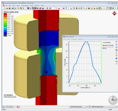
Simufact-GR-Simulationsmodell-und-simulierter-Presskräfteverlauf-Stufe2.png
