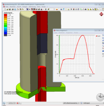
Simufact-GR-Simulationsmodell-und-simulierter-Presskräfteverlauf-Stufe-1.png
