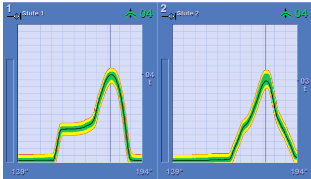
Simufact-GR-Prokos-gemessene-Presskraftverläufe.png
