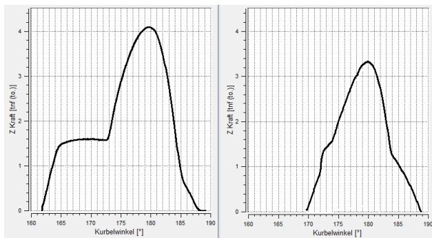
Simufact-GR-simulierte-Presskraftverläufe.png
