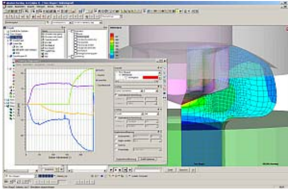
Bild 1: Simulation einer Schraubenherstellung in Simufact.forming 12
