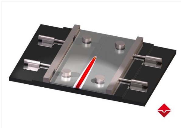
Bild 2: Simulation des Laserschweißens von Blechstrukturen in einer Spannvorrichtung
