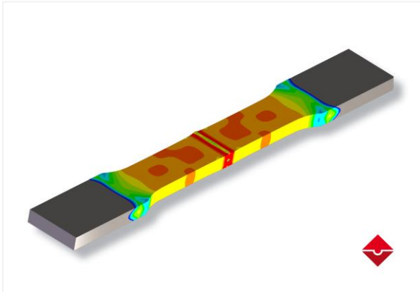
Bild 1: Simulation einer geschweißten Zugprobe - Schweißstrukturtest
